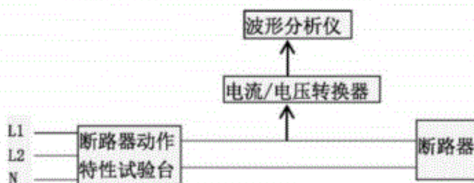
图 2 测量原理图
