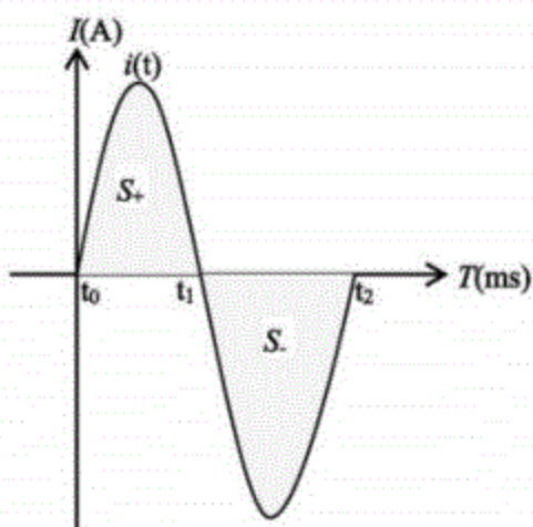
图3 正负半波面积差示意图
