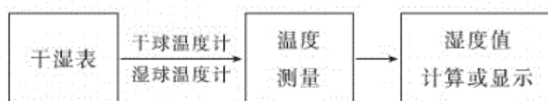
图 1 干湿表原理框图
