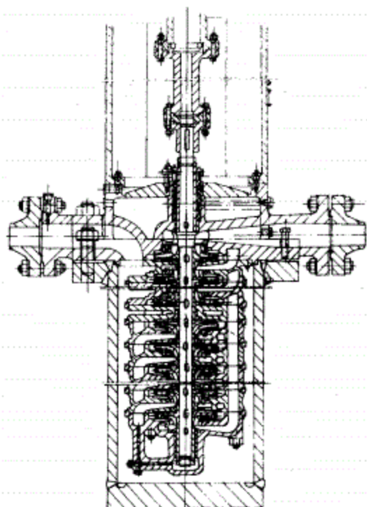
图10 立式筒式泵
