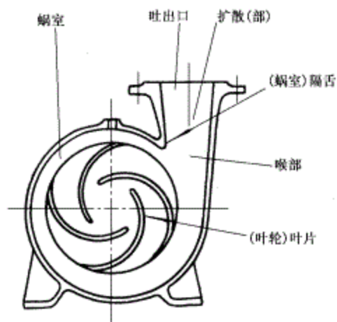
图 18 蜗形体
