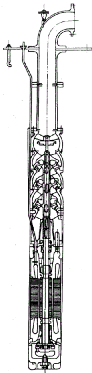
图11 潜水电泵
