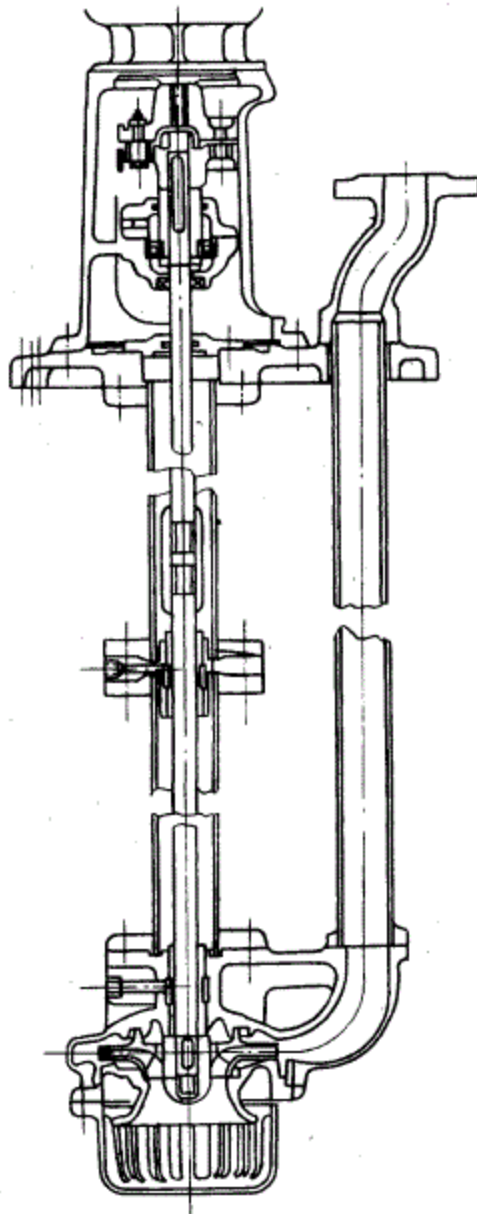
图 15 立式单吸蜗壳泵(液下式)
