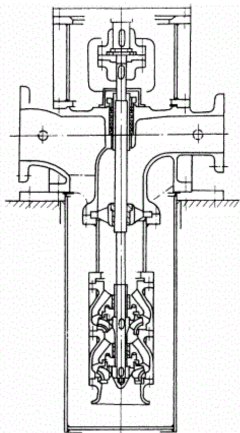
图9 地坑筒式泵
