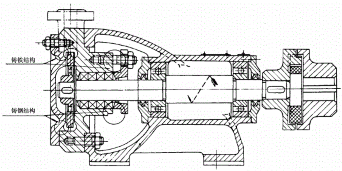
图1 一般单级旋涡泵
