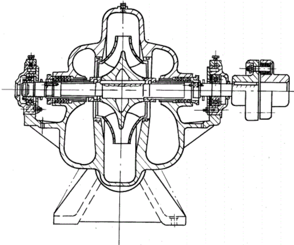
图3 卧式单级双吸泵(水平中开式)
