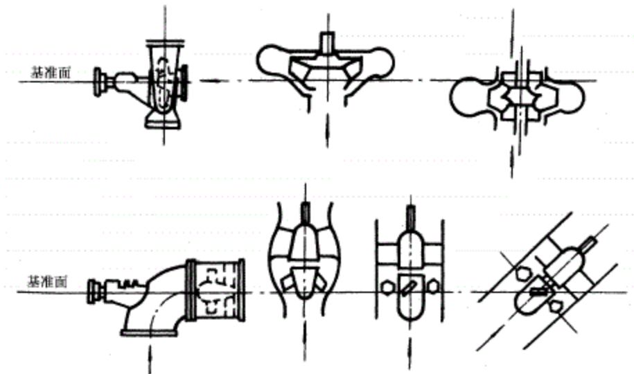
图 16 泵基准面
