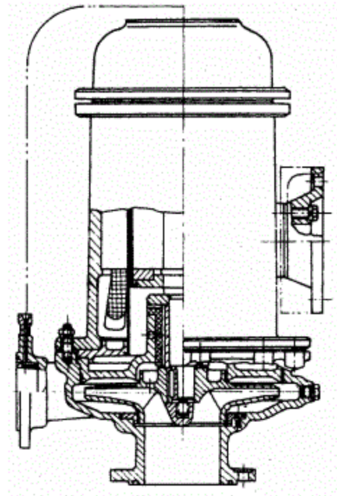
图8 屏蔽电泵
